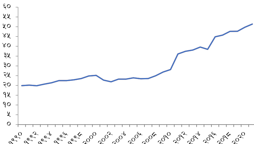
चार्ट १४(ख): नेपाल हरितगृह ग्यास उत्सर्जनको प्रवृत्ति (वार्षिक ग्यास उत्सर्जन दश लाख मेट्रिक टनमा)
