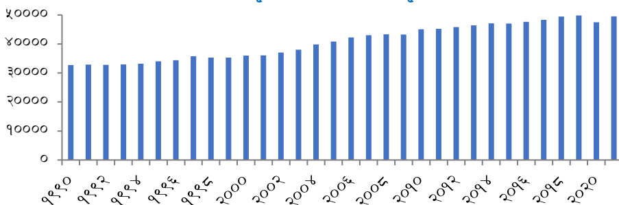
चार्ट १४(क): विश्वको हरितगृह ग्यास उत्सर्जनको प्रवृत्ति (दशलाख टन CO 2 )
