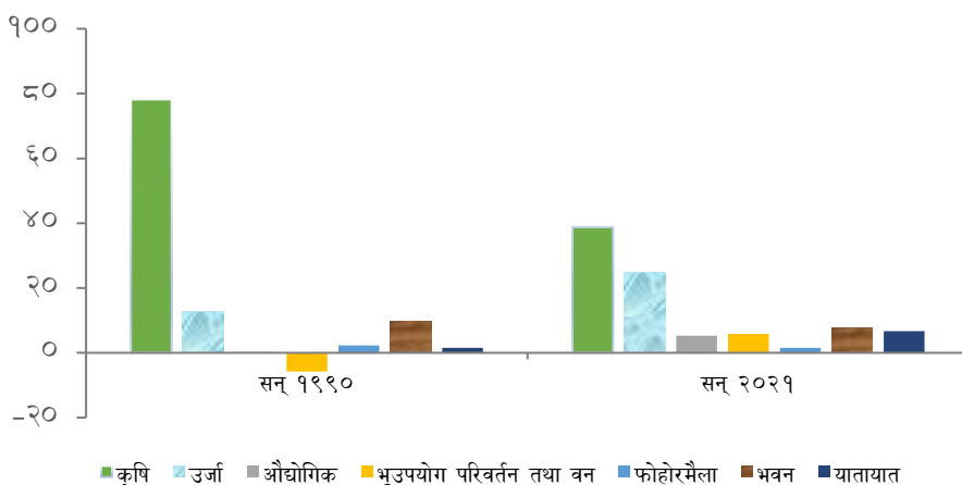
चार्ट १४(ग): क्षेत्रगत हरित ग्यास उत्सर्जन (प्रतिशतमा)
